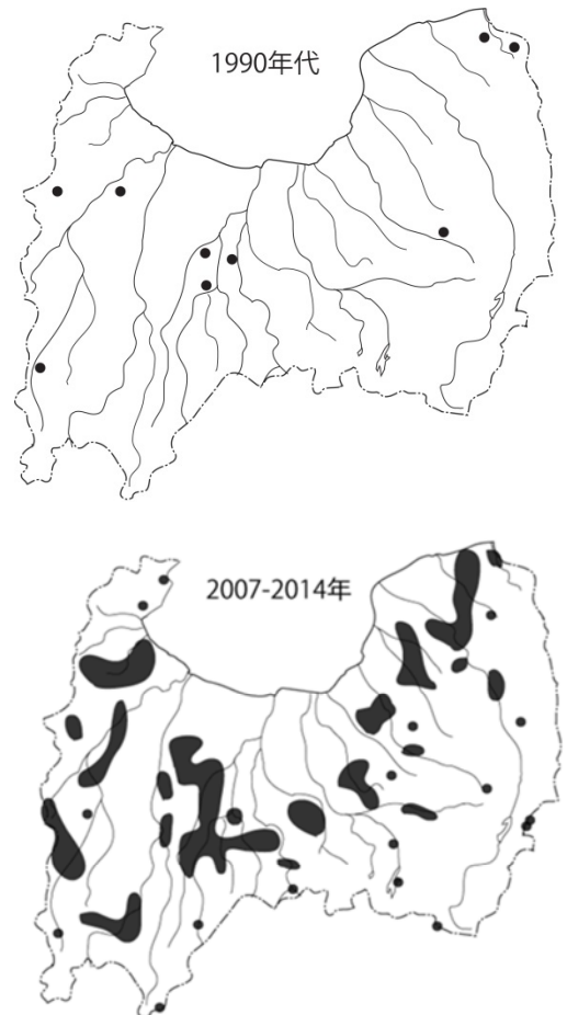
図2. 富山県のニホンジカの分布の変化(上 南部(1997)より,下 富山県動物生態研究会(2015),中部森林管理局富山森林管理署(2014,2015)より作図)。
