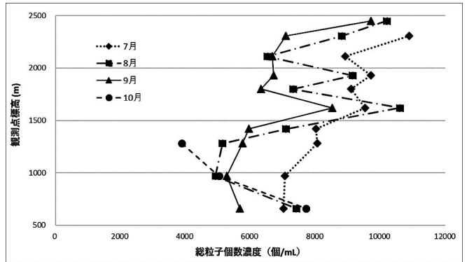
図9 各月の総粒子個数濃度の高度分布。
