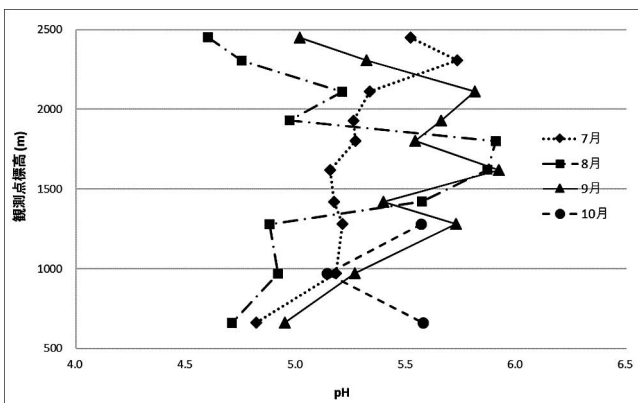
図8 各月のpHの高度分布。
