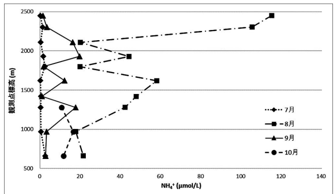
図6 各月の \text{NH}_4^+ 濃度の高度分布。
