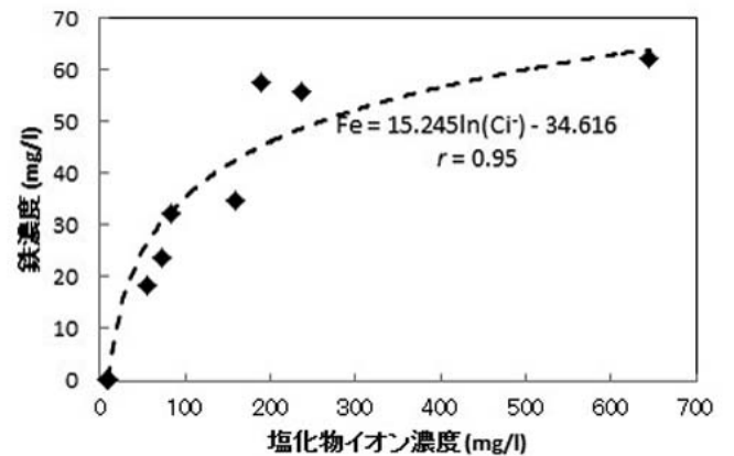
図7 四方地区の井戸水の塩化物イオン濃度と鉄濃度との関係
