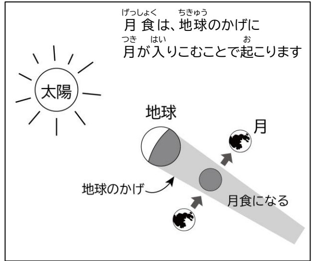
図2 月食とは
